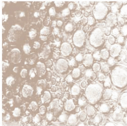
Öl-Wasser Struktur
